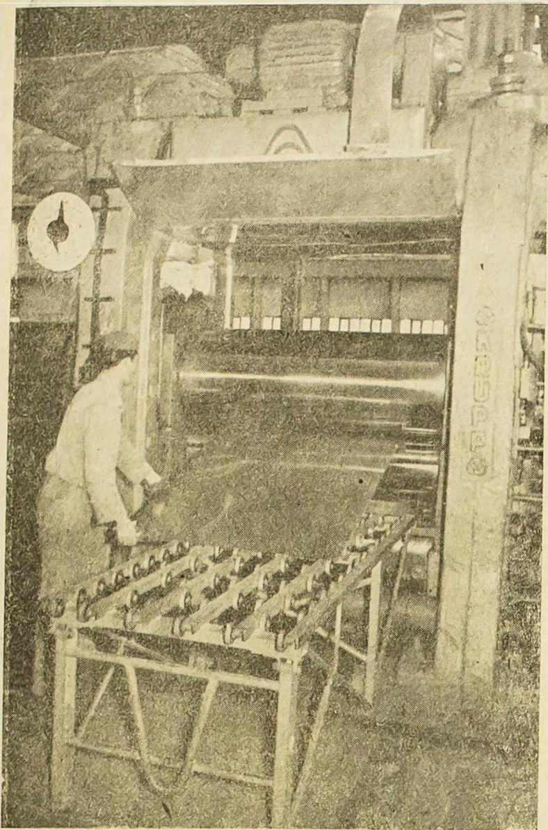
TLM »Boris Kidrič« Valjanje aluminija
