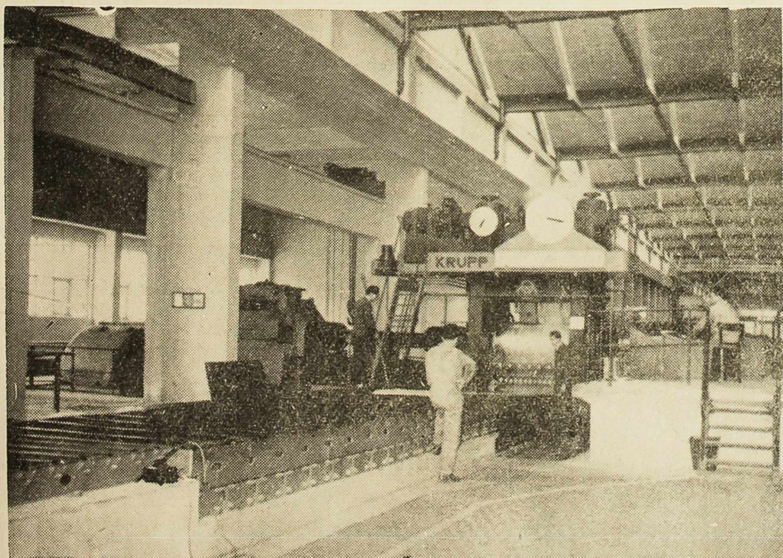
TRIO-STAN NA KOJEM SE OBAVLJA VALJANJE ZAGRIJANI H ALUMINIJSKIH BLOKOVA
