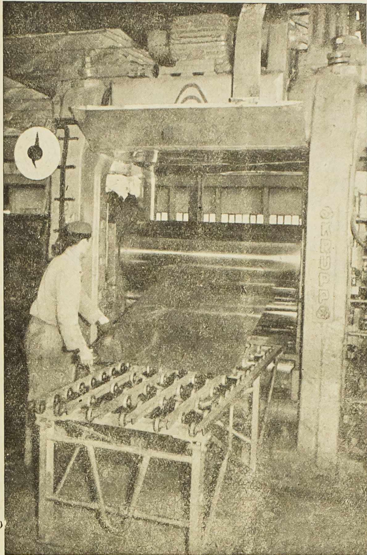
ZAVRŠNA FAZA U PROCESU VALJANJA LIMA
