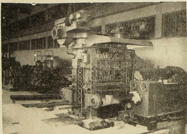
MODERNI TIP VALJAČKOG STANA ZA IZRADU ALUMINIJSKIH LISTICA (FOLIJA)
