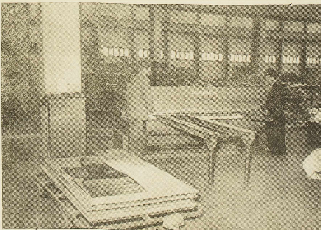
REZANJE IZVALJANOG LIMA NA KONAČNI FORMAT
