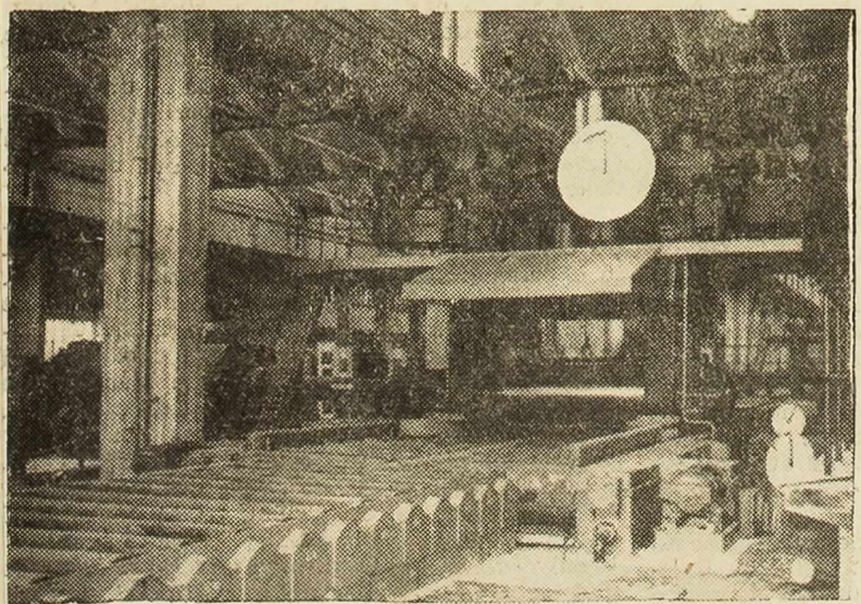
STROJ ZA IZRADU ALUMINIJSKE TRAKE
