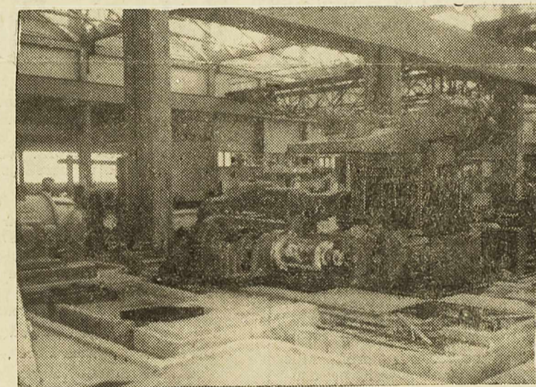
NAJMODERNIJI TIP STROJA ZA VALJANJE TRAKA
